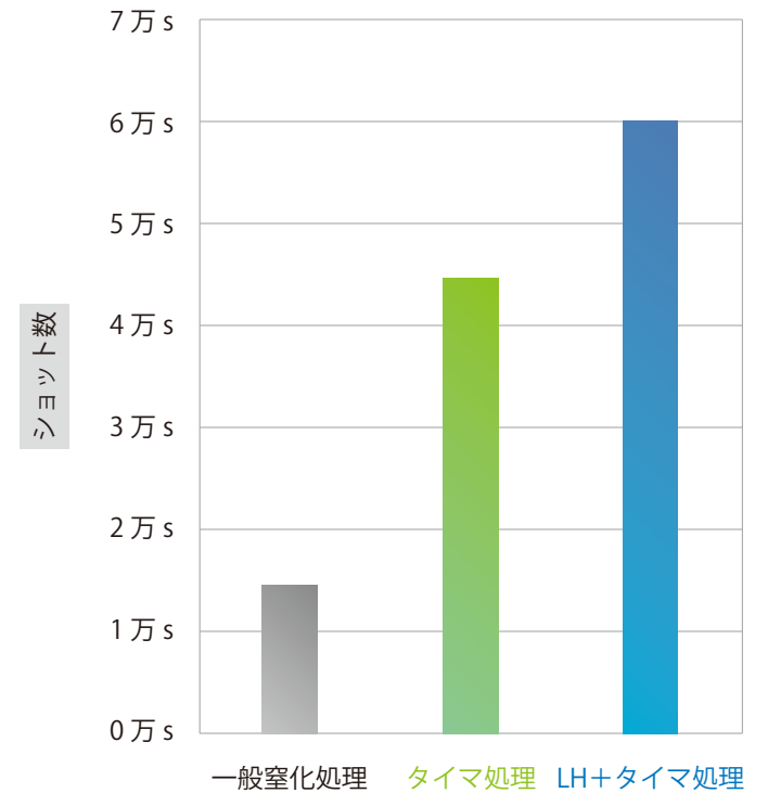
【ヒートチェック寿命の比較】
