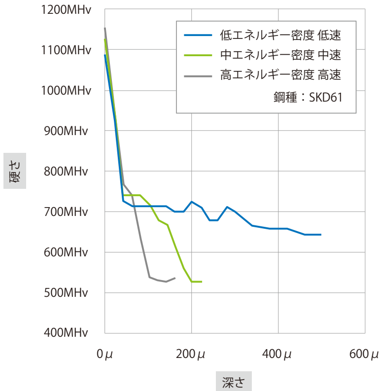
【レーザー焼入れ+タイマ処理後の断面硬さ分布】
